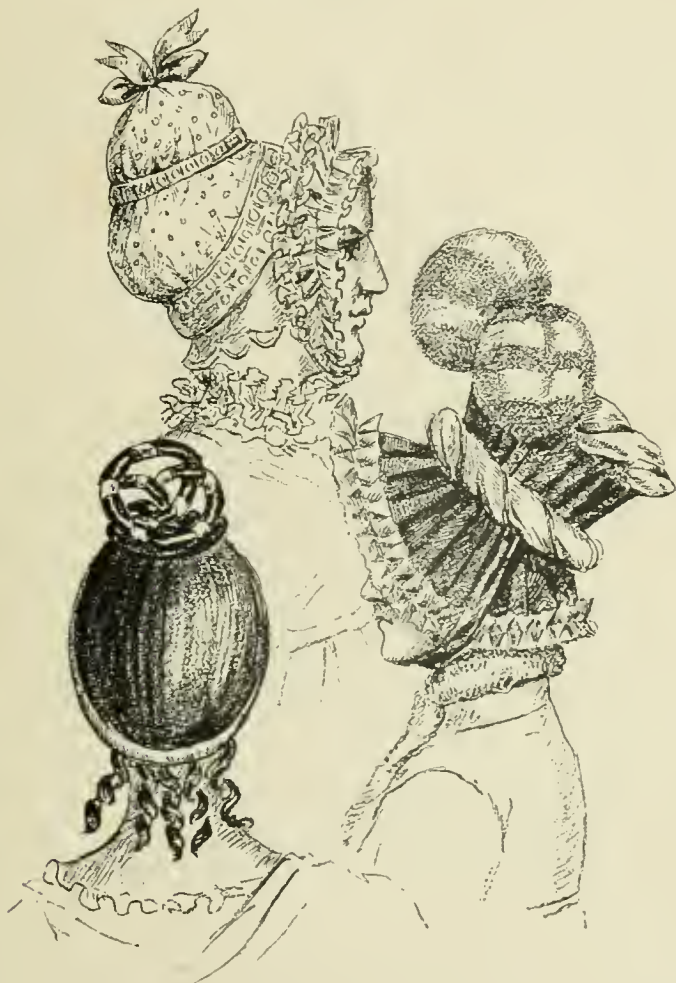
Fig. 544. — Modes de 1820.
